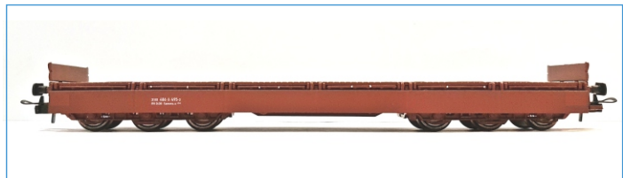
6-achsiger Schwerlastwagen Bauart Samms-u 454 der DB AG (Epoche V) braun, mit abgeklappten Bordwänden, 1. Betriebsnummer NW 52055 DC 2L TT 54,90 €
