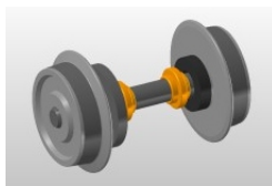
NZ 22128 Antriebsradsatz V45 mit Haftreifen u. Lager- schalen für 2L GS 7,65 €
