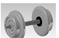
NZ 33280 Scheibenradsatz 10 mm, zapfengelagert einseitig isoliert
